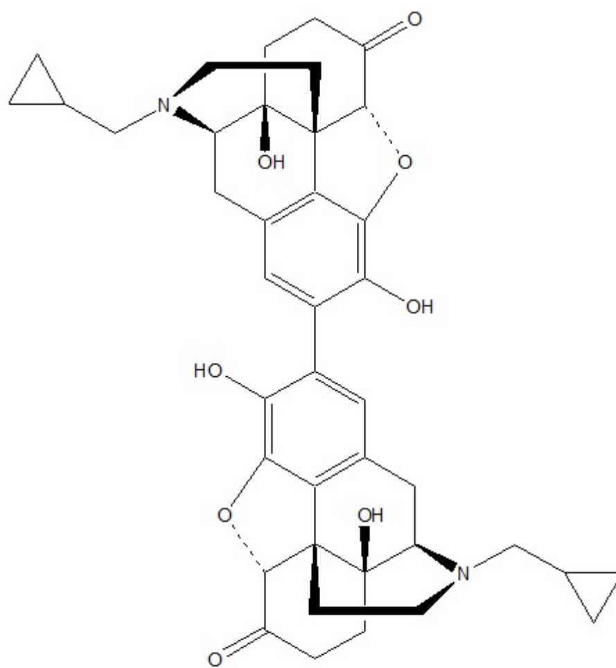
2,2'-Bisnaltrexone
